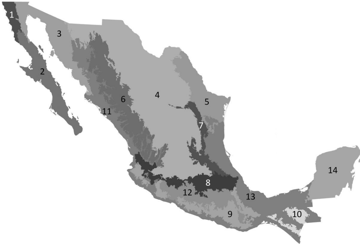
Figura 26. Provincias biogeográficas de México, modificado de Morrone et al. , 2017. Provincias Neárticas: 1) Provincia californiana, 2) Provincia bajacaliforniana, 3) Provincia sonorese, 4) Provincia del desierto de Chihuahua, 5) Provincia de Tamaulipas; Provincias intermedias (Neártica-Neotropicales): 6) Provincia de la Sierra Madre Occidental, 7) Provincia de la Sierra Madre Oriental, 8) Provincia del Cinturón Volcánico Transmexicano, 9) Provincia de la Sierra Madre del Sur, 10) Provincia de las tierras altas de Chiapas; Provincias Neotropicales: 11) Provincia de tierras bajas del Pacífico, 12) Provincia de la cuenca del Balsas, 13) Provincia veracruzana, 14) Provincia de la Península de Yucatán.
